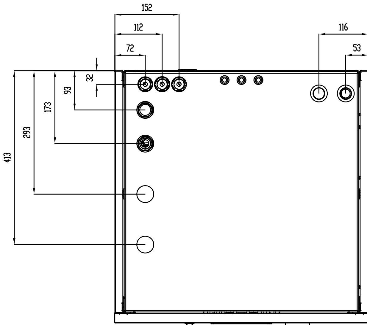
Slika 3.2: Pozicije priključaka
