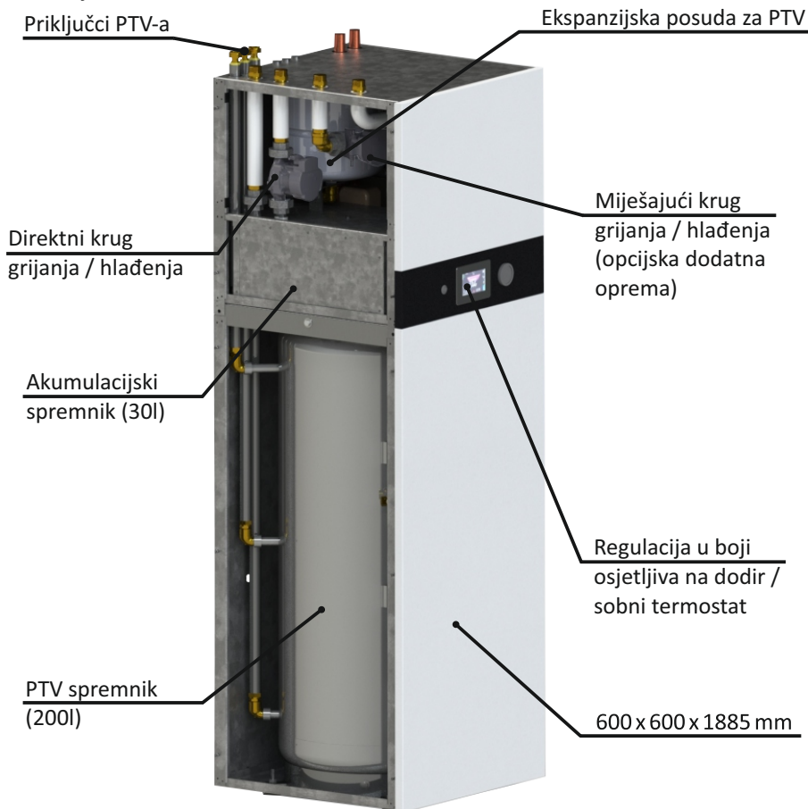
Slika 5.1: Dijelovi Tower-M/200
