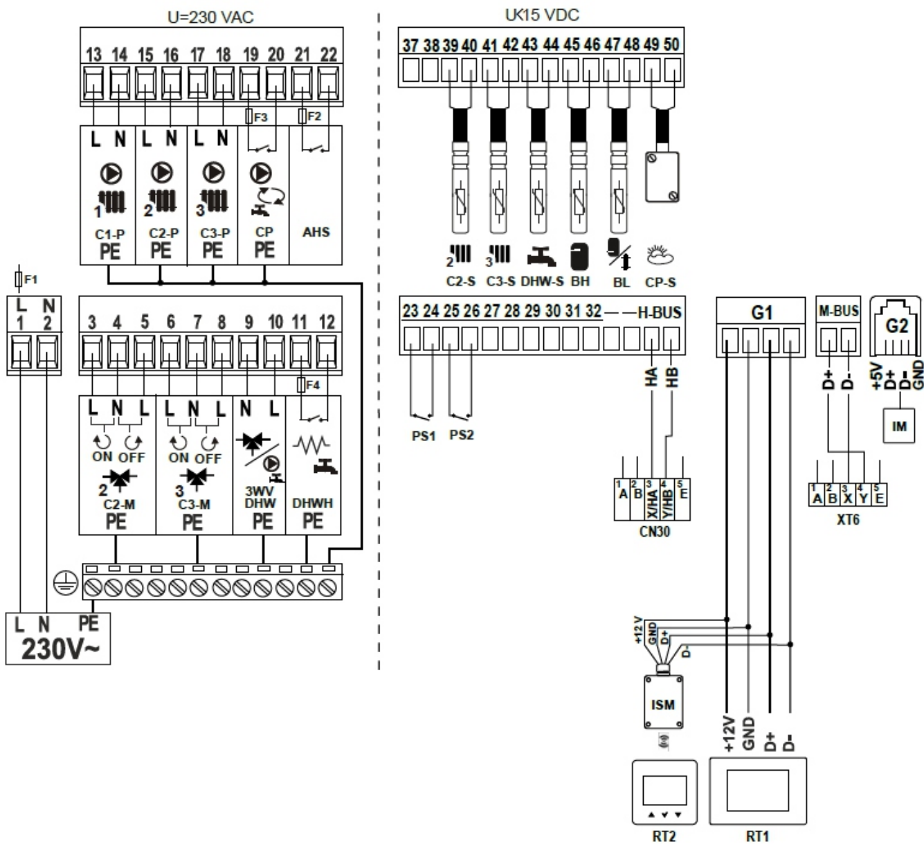
Slika 4.1: Električna shema
