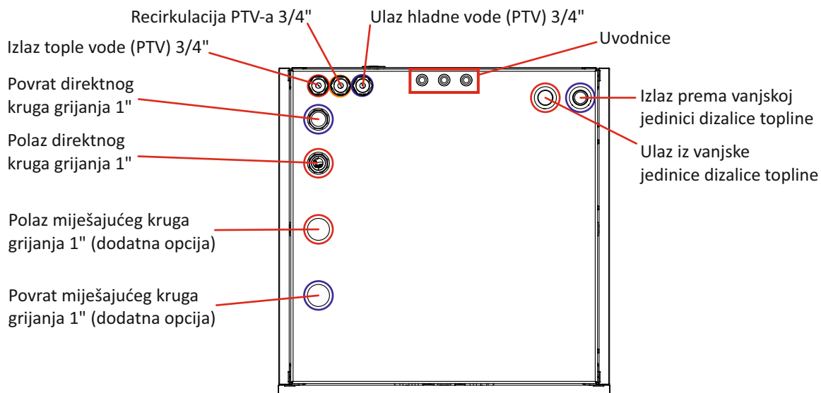
Slika 5.2: Tlocrt Tower-M/200 jedinice s prikazanim priključcima
