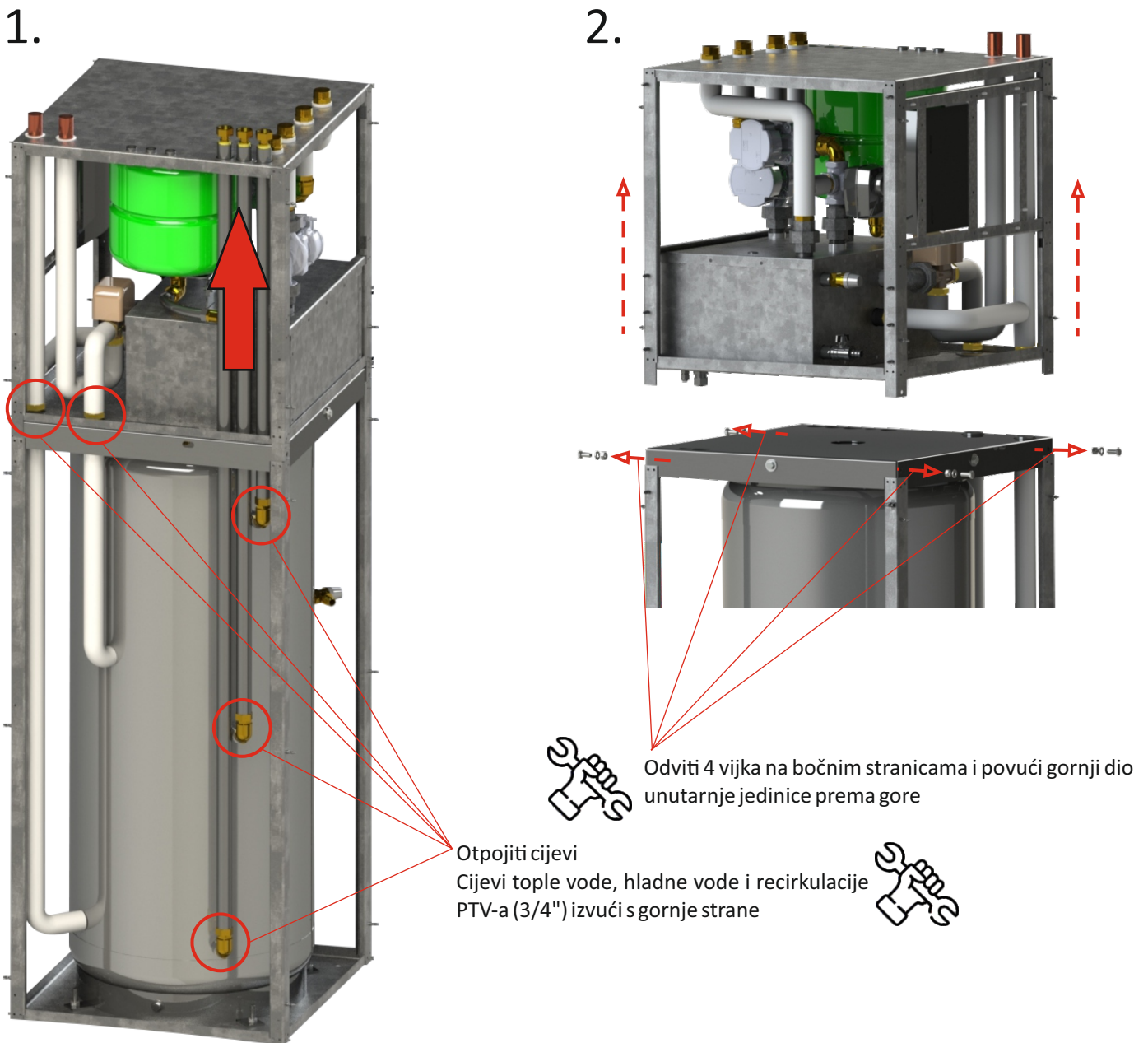
Slika 5.3: Rastavljanje Tower-M/200 jedinice na dva dijela
