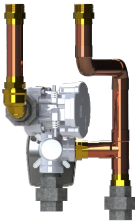
Slika 5.4: Ugradnja dodatnog miješajućeg kruga za Tower-M/200
