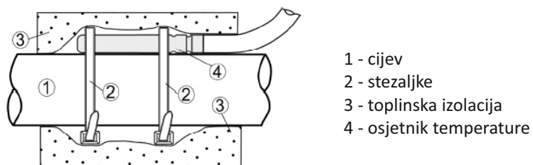
Slika 5.5: Ugradnja osjetnika topline dodatnog kruga
