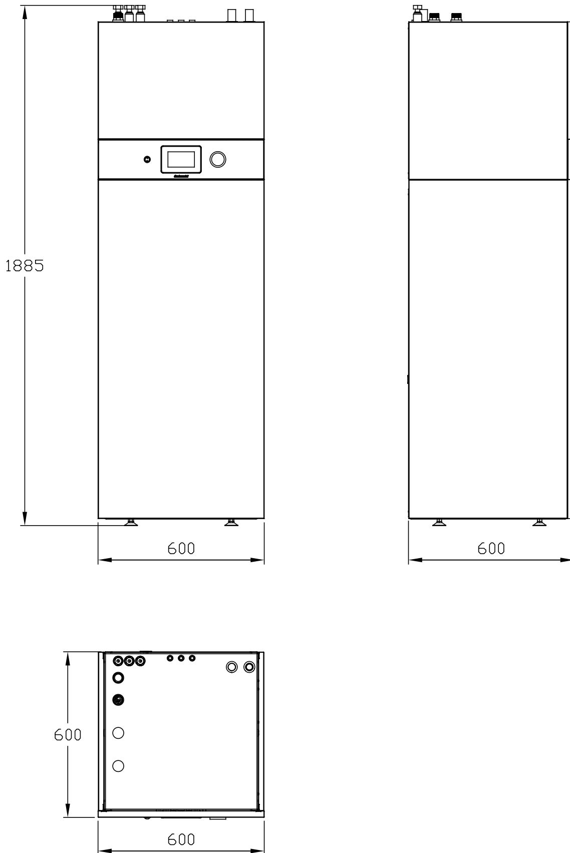
Slika 3.1: Dimenzije Tower-M/200 (jedinice: mm)
